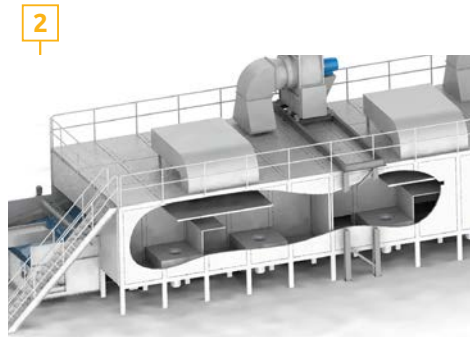
Cámara TopDown dirección del aire a través de la banda de abajo hacia arriba Vista de la estación de transferencia
