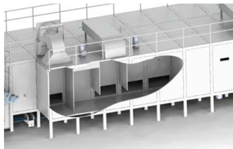
Cámara BottomUP dirección del flujo de aire a través de la banda de arriba a abajo
